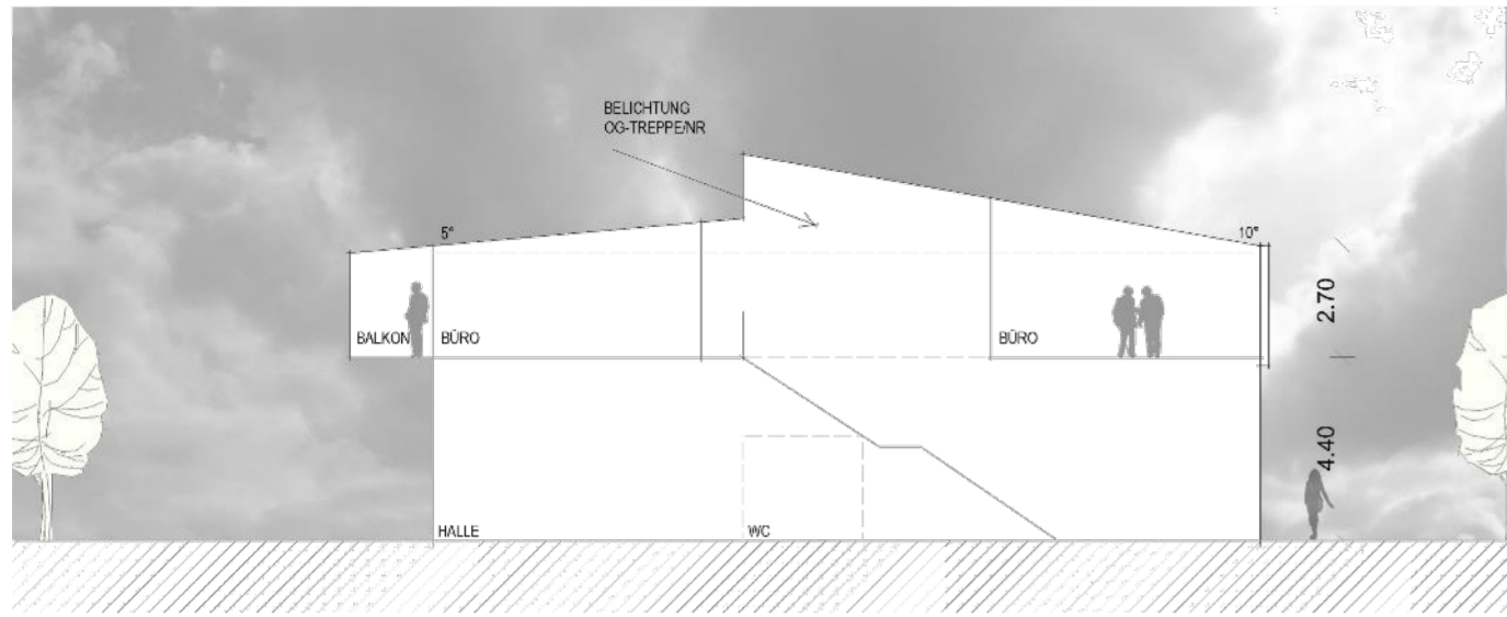
SCHNITT 1:200
